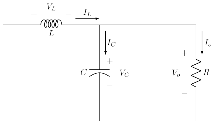
Figura 6 – Circuito equivalente com a chave aberta
